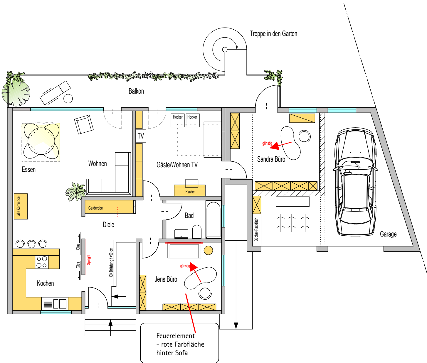
Grundriss EG - Lösungskonzept - M 1 : 100
